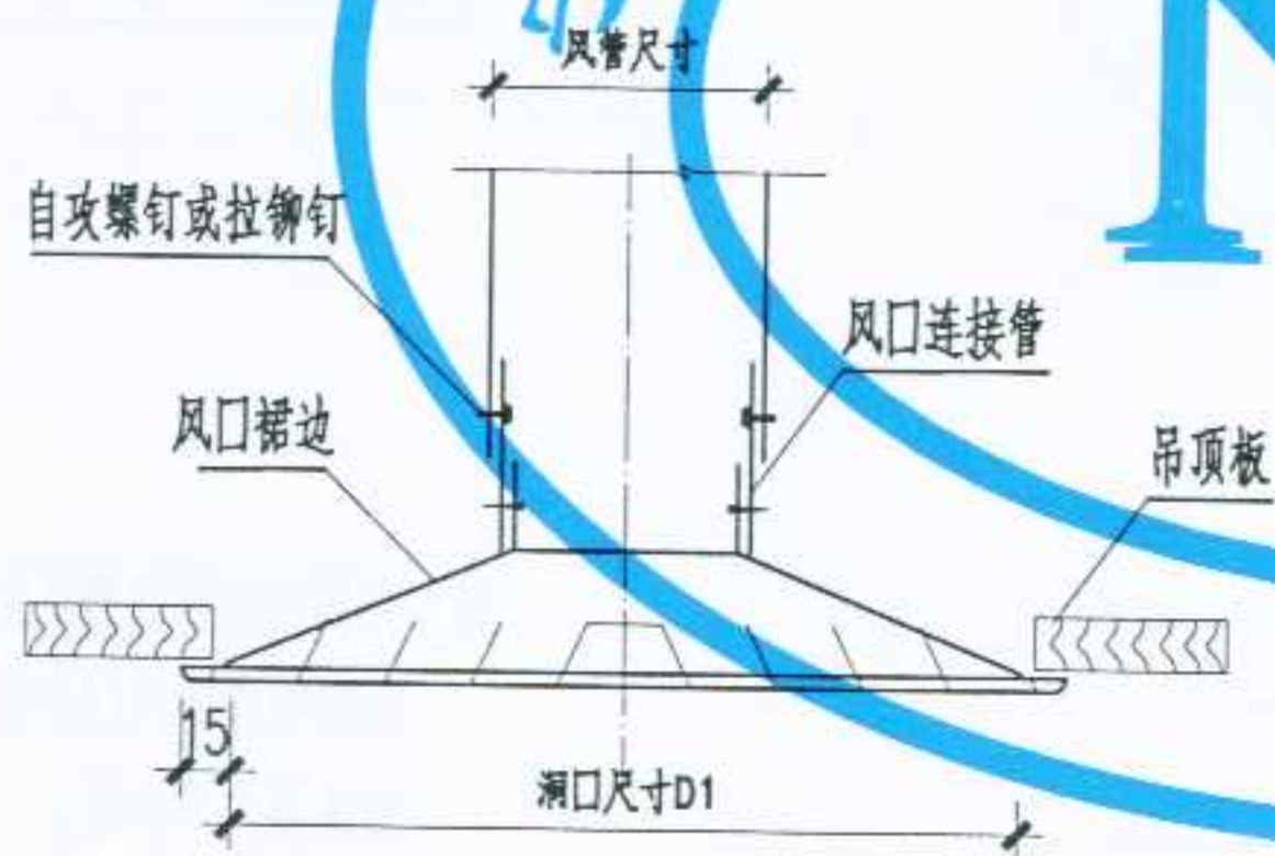
圆形散流器与风道固定式安装法
