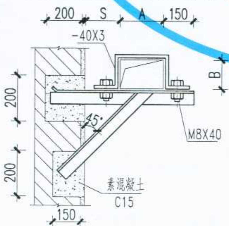
矩形不保温风管墙上斜撑支架
