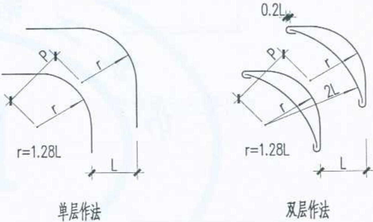
直角矩形弯管内导流叶片的设置
