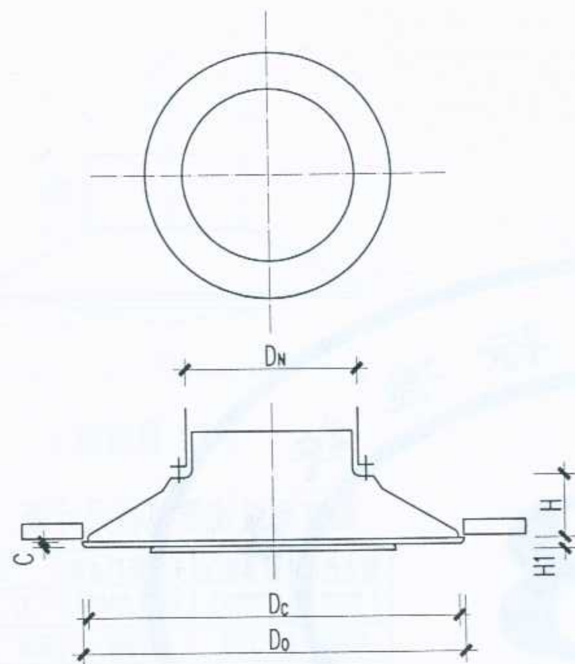
YS(水平贴附型)
