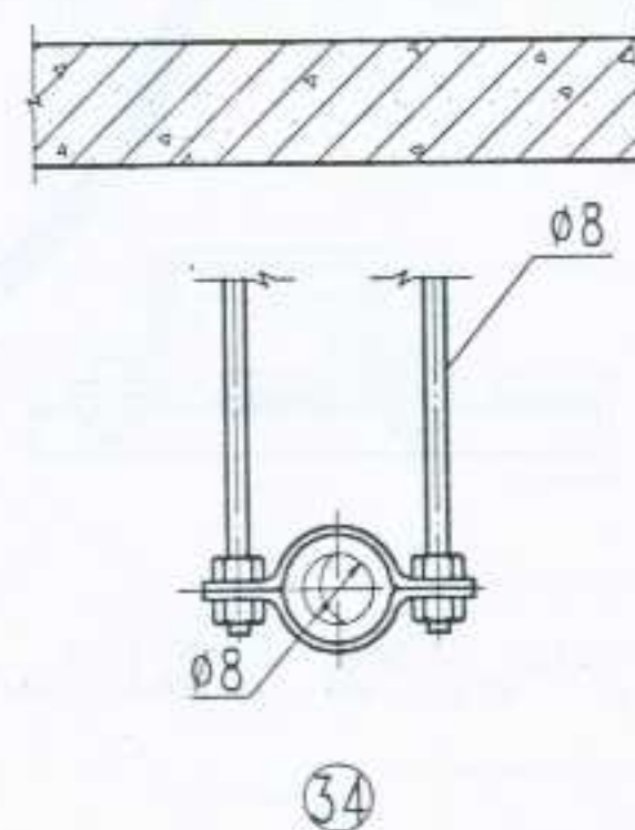
圆形保温风管双杆吊架
