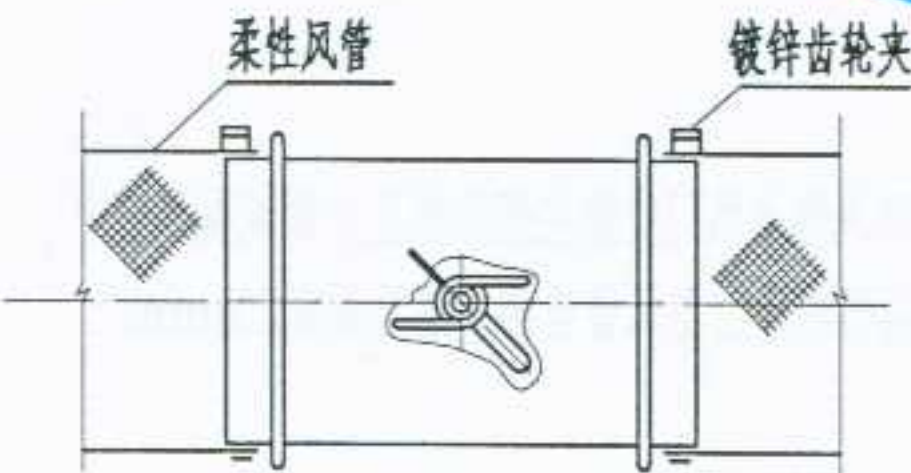
小风门与柔性风管连接
