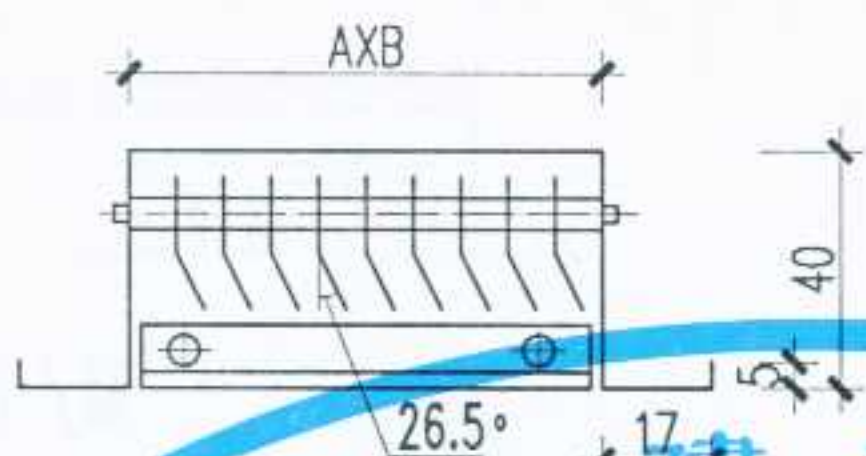
双层固定百叶
