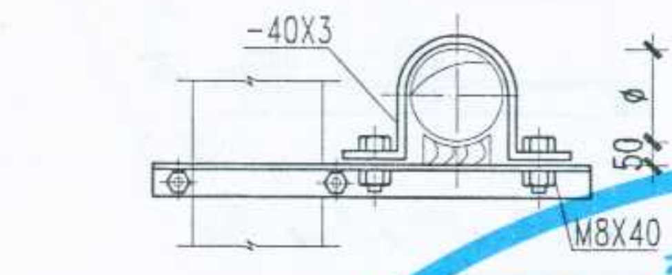
圆形不保温风管柱上支架(一)
