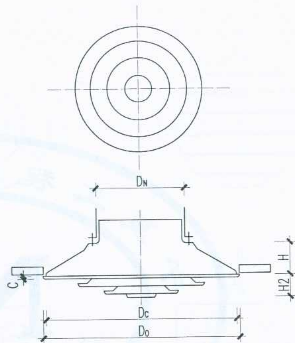
YS(凸形水平型)
