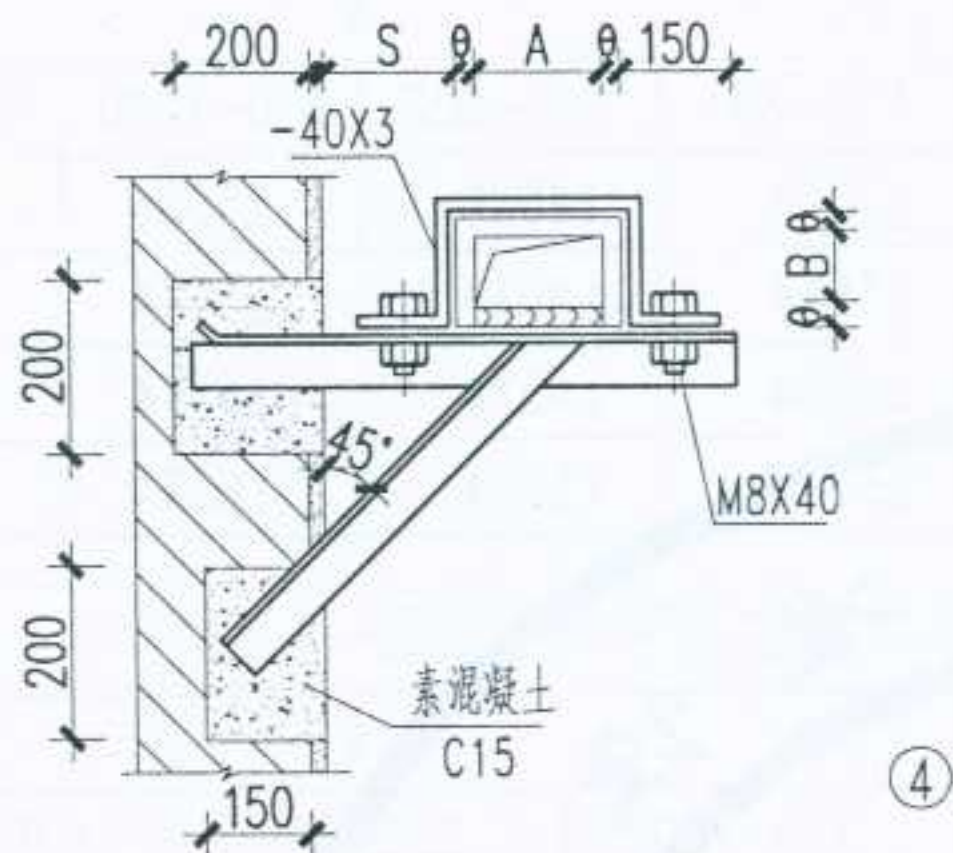
矩形保温风管墙上斜撑支架
