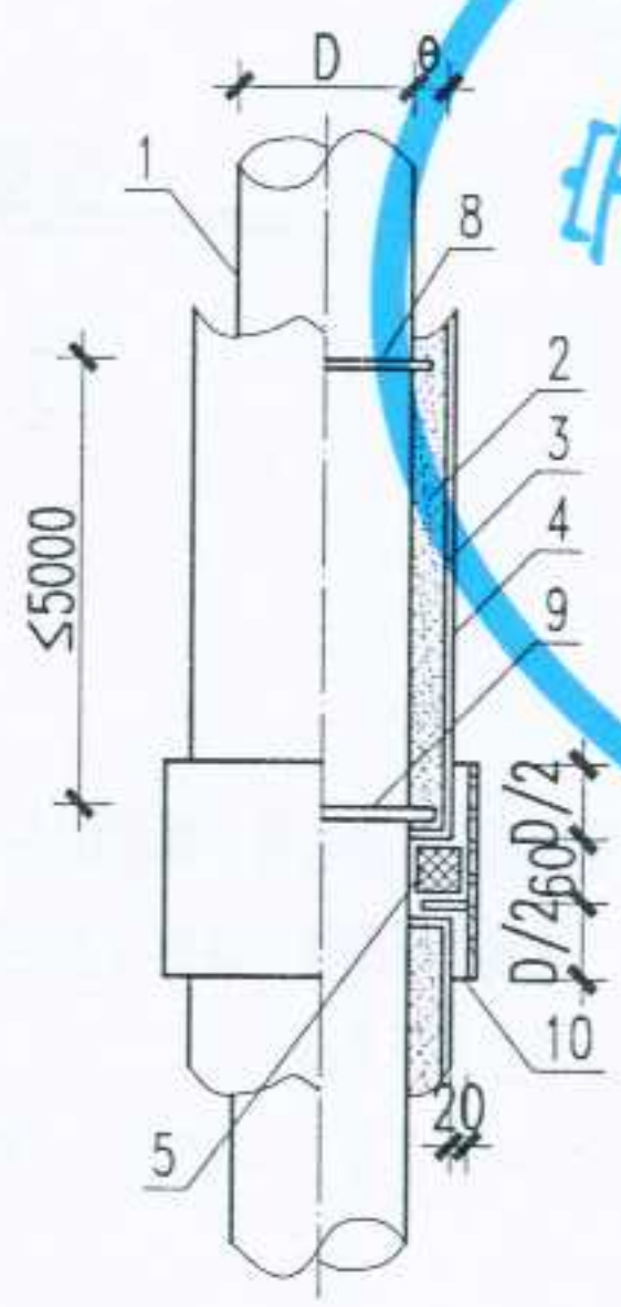
垂直管道保温结构
