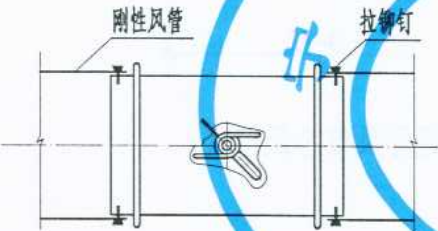
小风门与刚性风管连接
