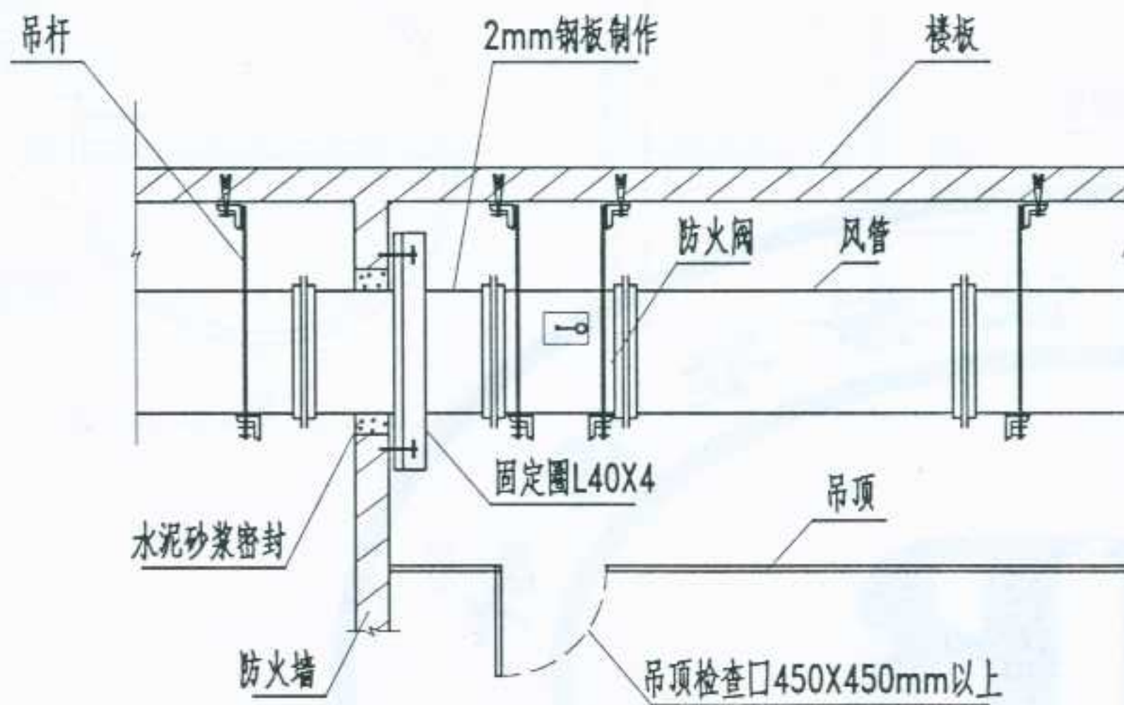
风管水平穿越防火分区隔墙时防火阀的安装
