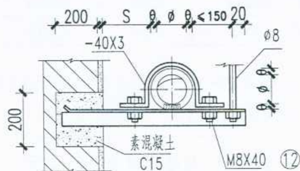
圆形保温风管墙上支吊架
