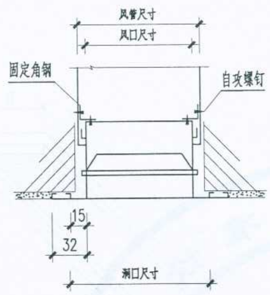
风管插入安装法
