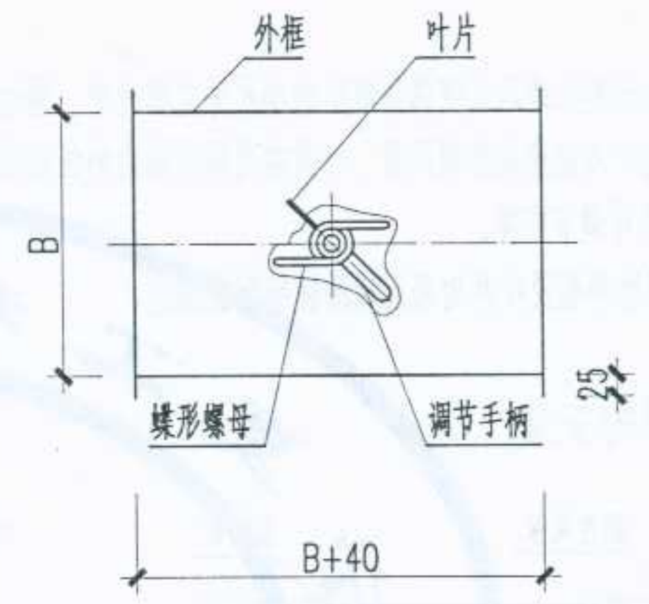
矩形风管小风门
