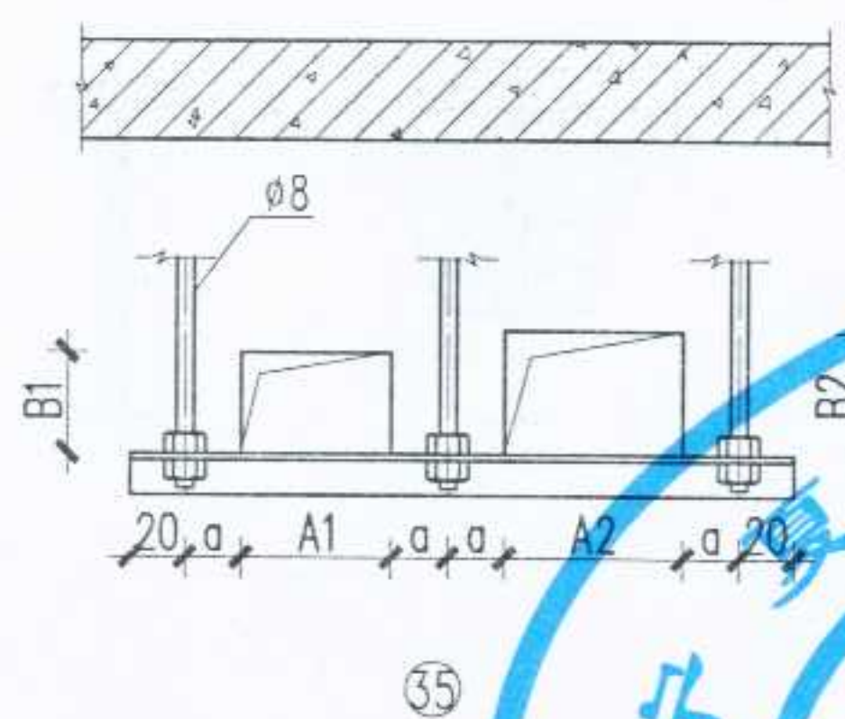
矩形不保温风管平行三杆吊架
