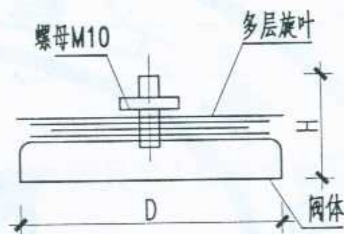
旋叶式圆形风阀
