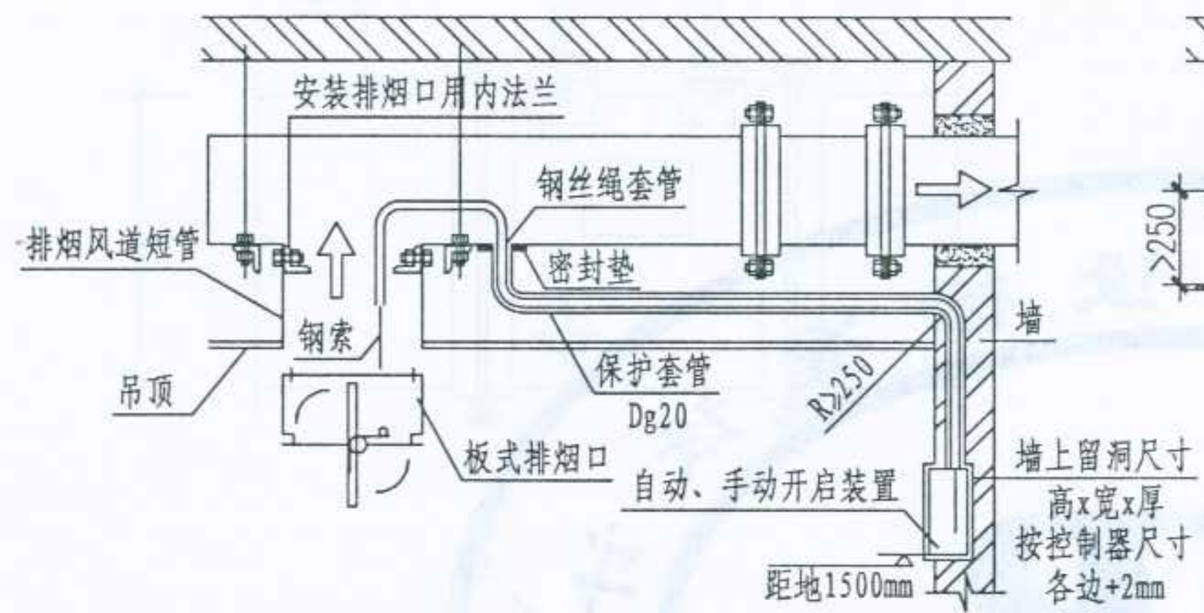
排烟口安装示意图
