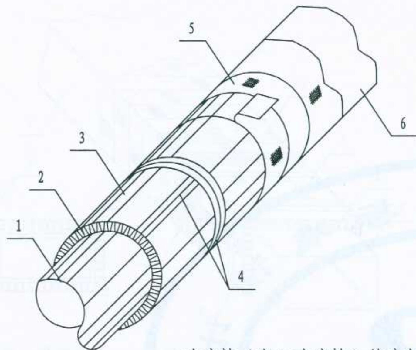
玻璃棉（离心玻璃棉）管壳保温
