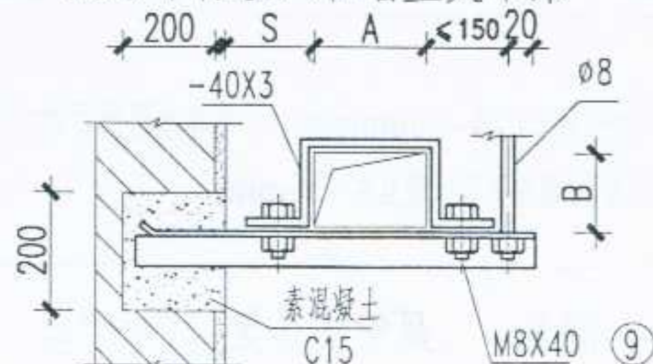
矩形不保温风管墙上支吊架
