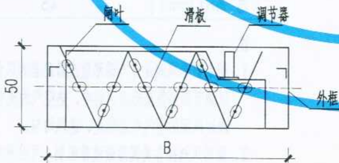
单层叶片钢制人字风阀
