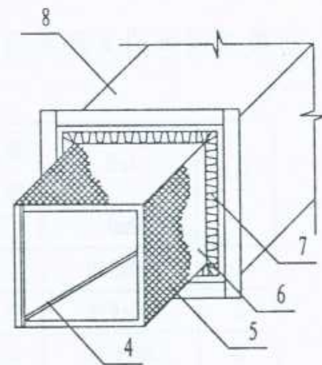
节点构造
