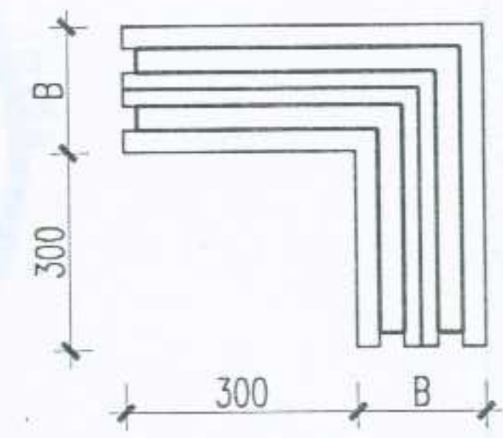
角形段
