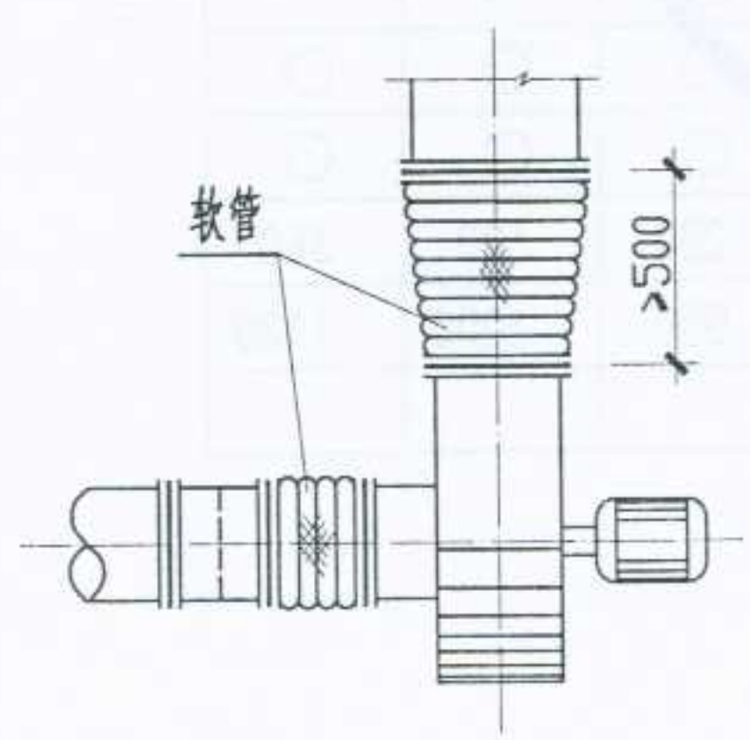
风机与风管间连接示意
