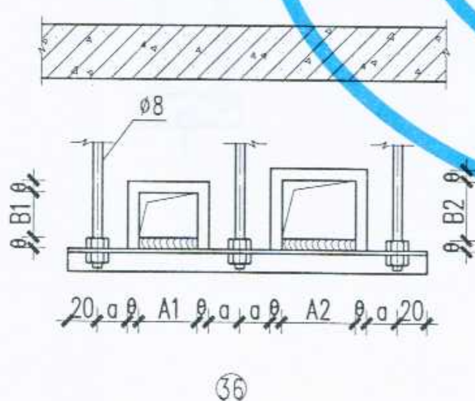
矩形保温风管平行三杆吊架
