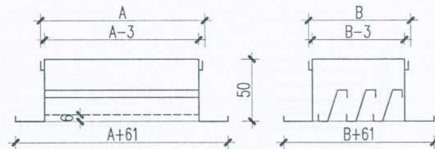
钢/不锈钢防水百叶风口
