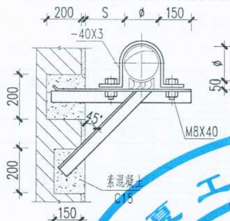
圆形保温风管墙上斜撑支架
