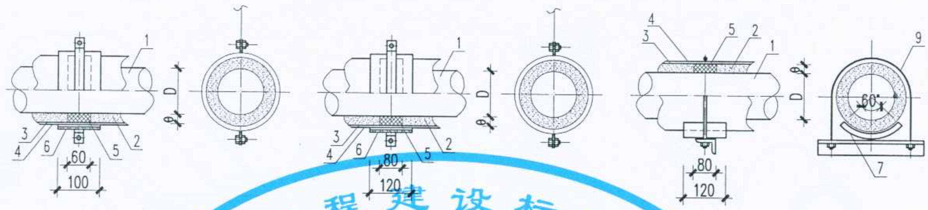
DN ≤ 100mm 管道吊架保温结构
