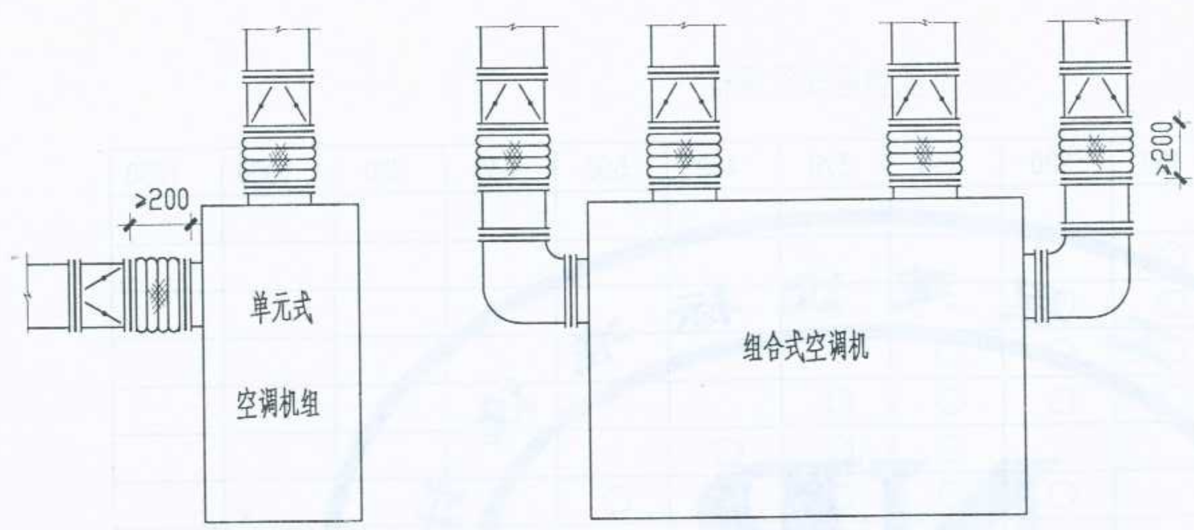
单元式空调机组、组合式空调机与风管间连接示意
