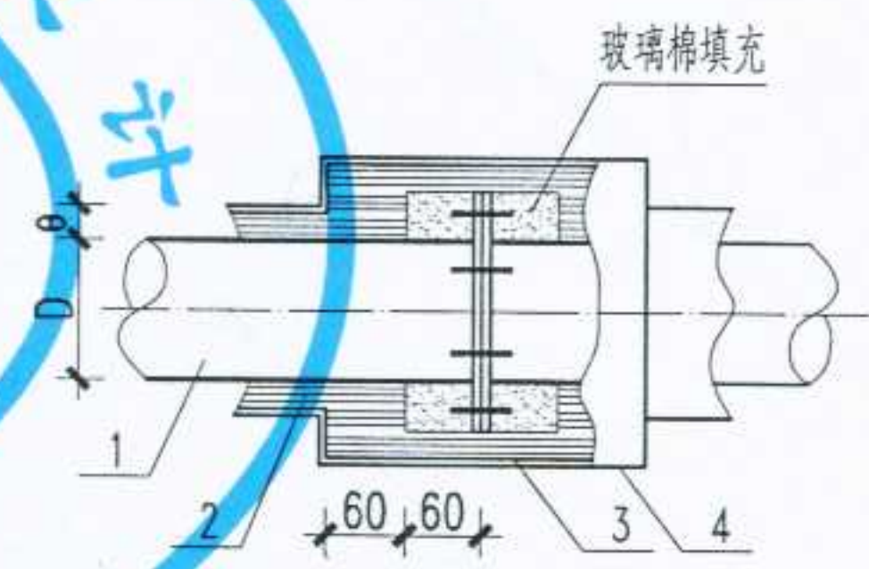
法兰保温结构
