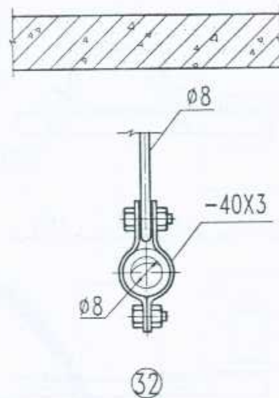
圆形保温风管单杆吊架
