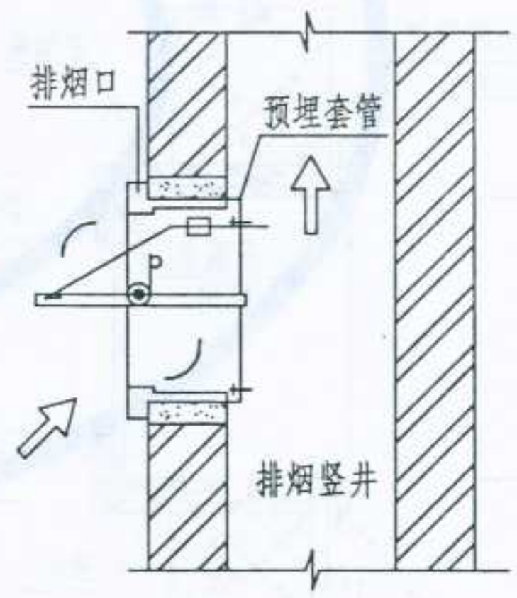
板式排烟口在竖井墙上安装
