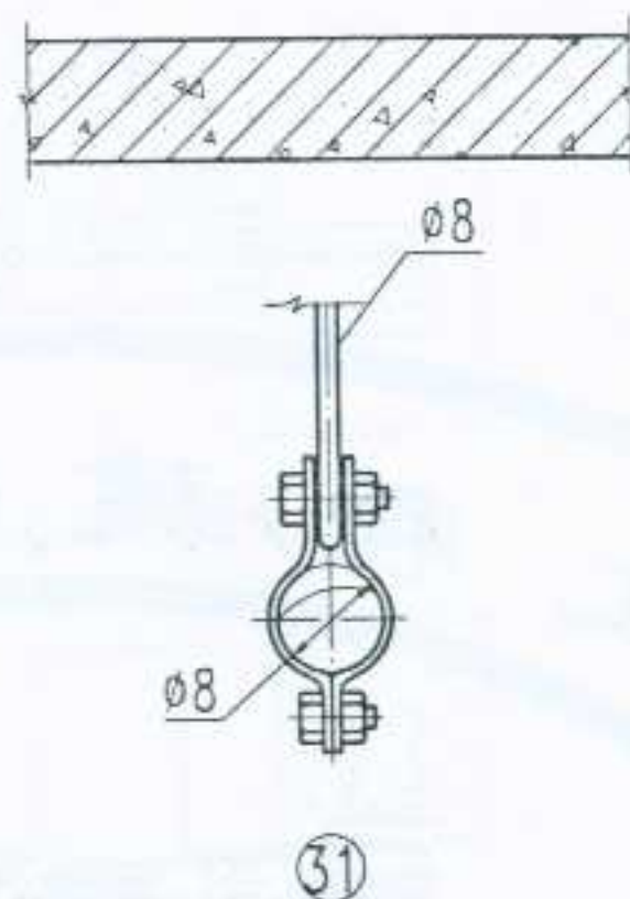
圆形不保温风管单杆吊架
