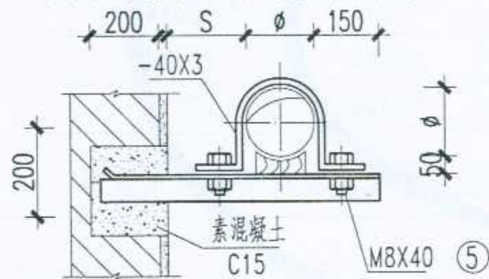
圆形不保温风管墙上支吊架
