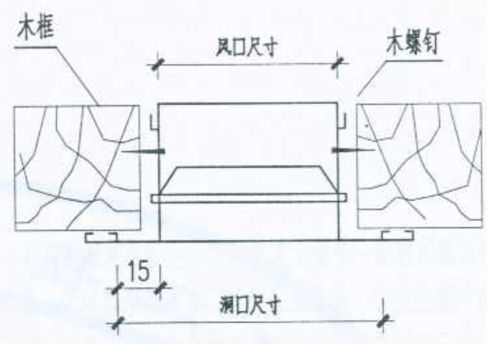
外门框安装法 (一)
