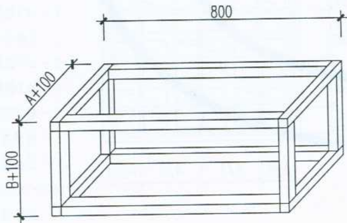
木框示意
