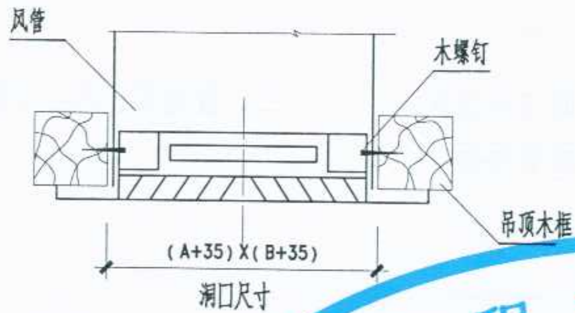
方形散流器叶片与边框固定式安装法
