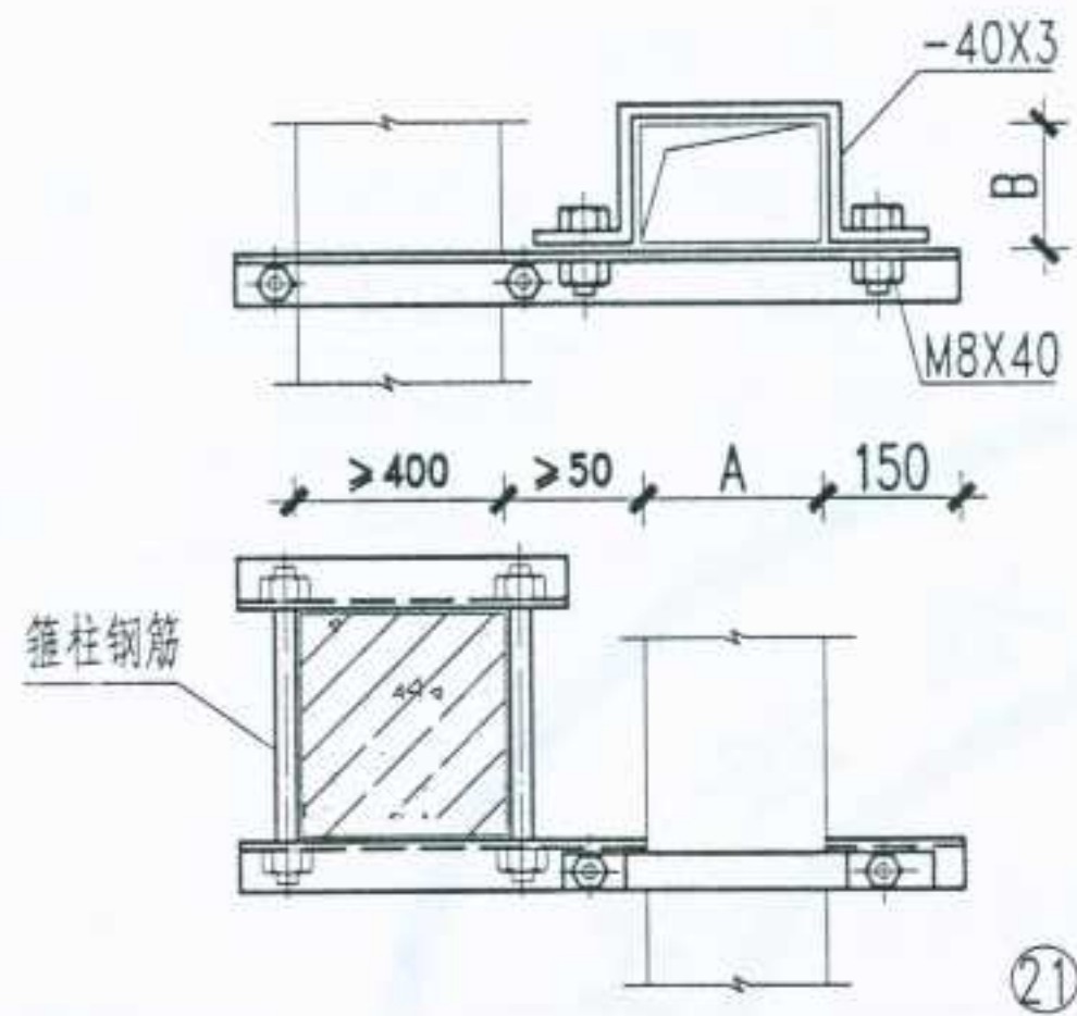
矩形保温风管柱上支架(二)
