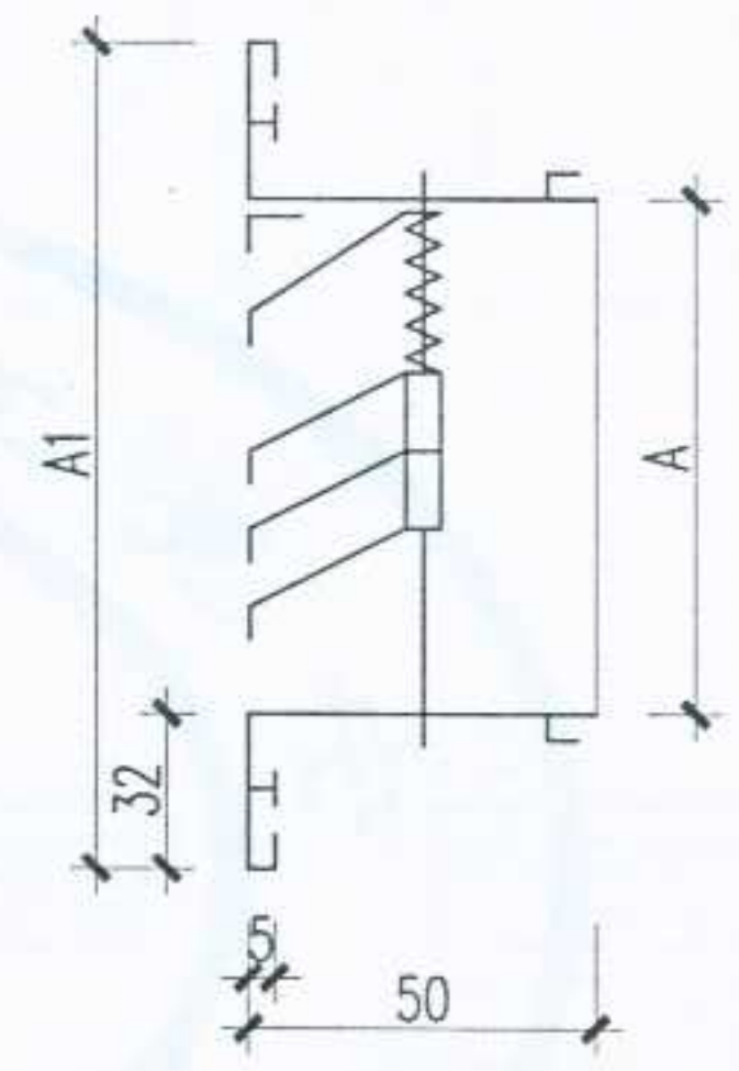
TF (活芯式)
