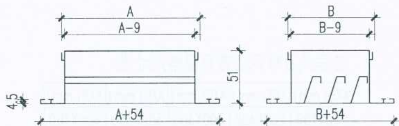
铝制防水百叶风口
