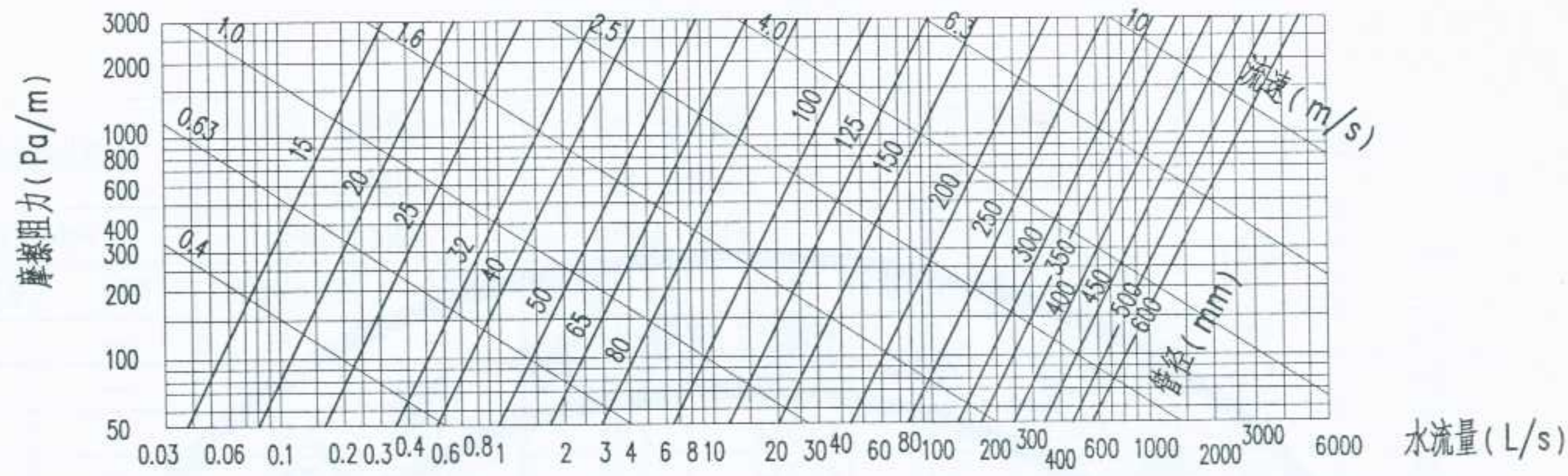
钢管的水摩擦阻力损失
