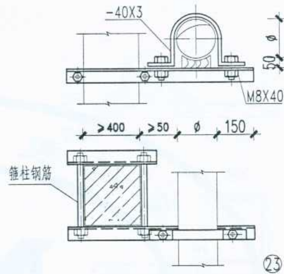
圆形不保温风管柱上支架(二)
