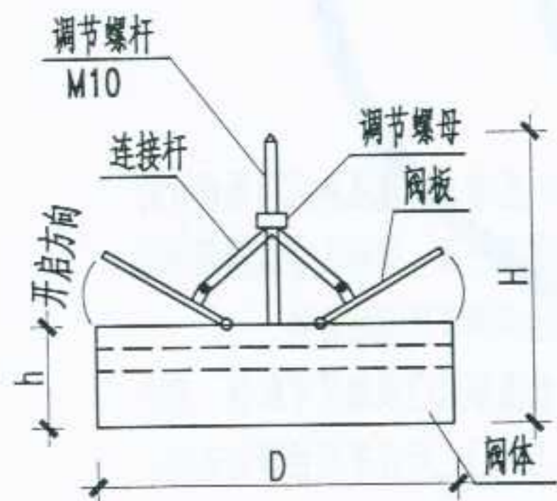
双向圆形风阀
