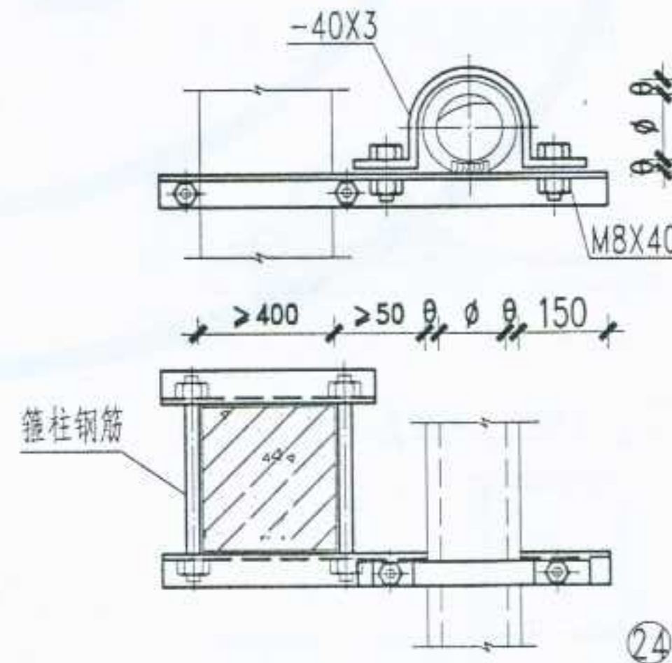
圆形保温风管柱上支架(二)
