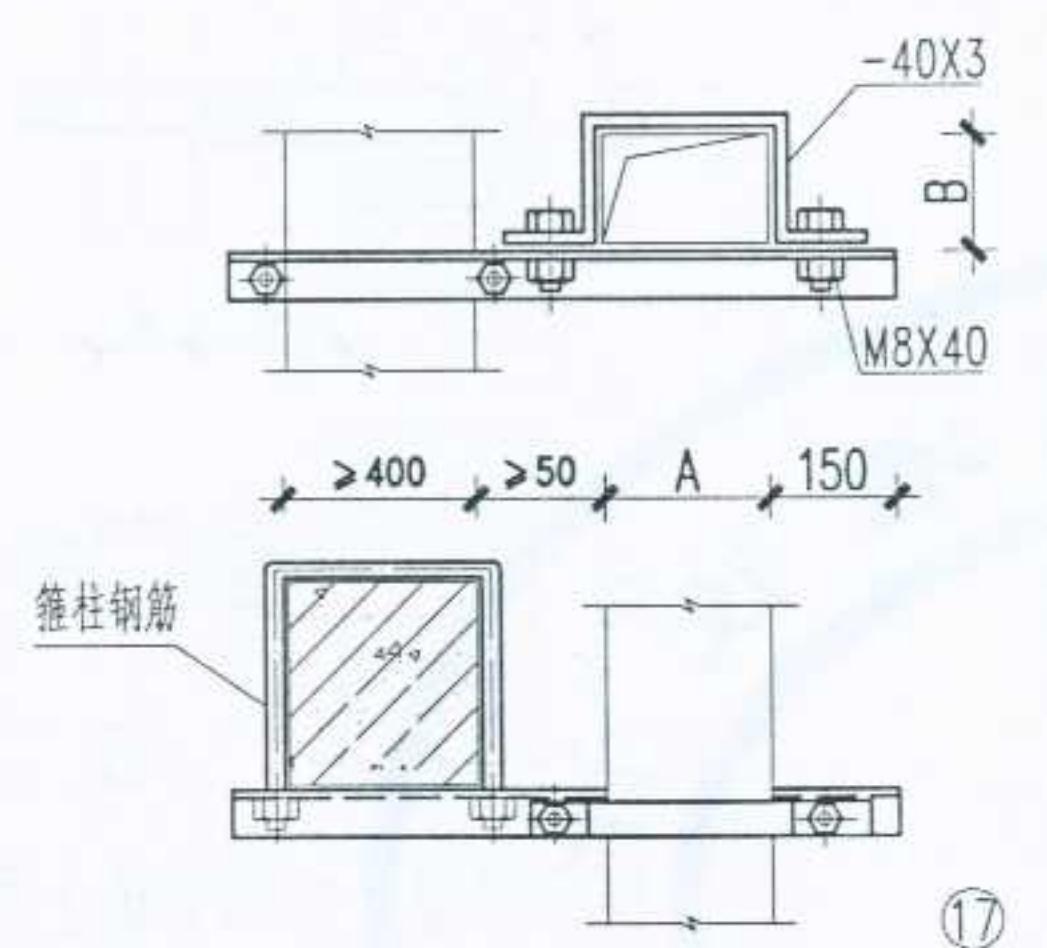
矩形不保温风管柱上支架(一)
