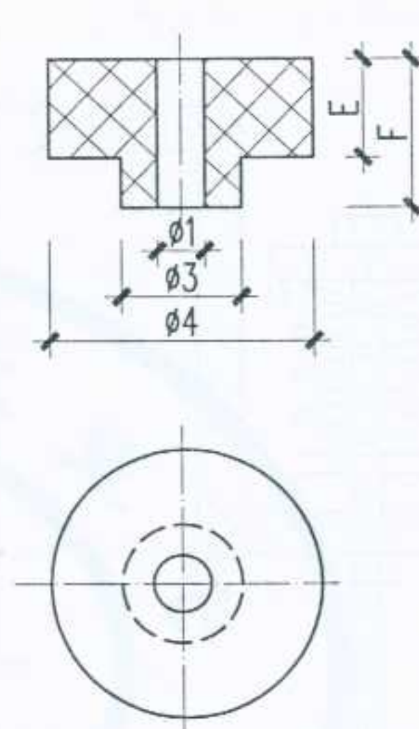
橡胶减振器
