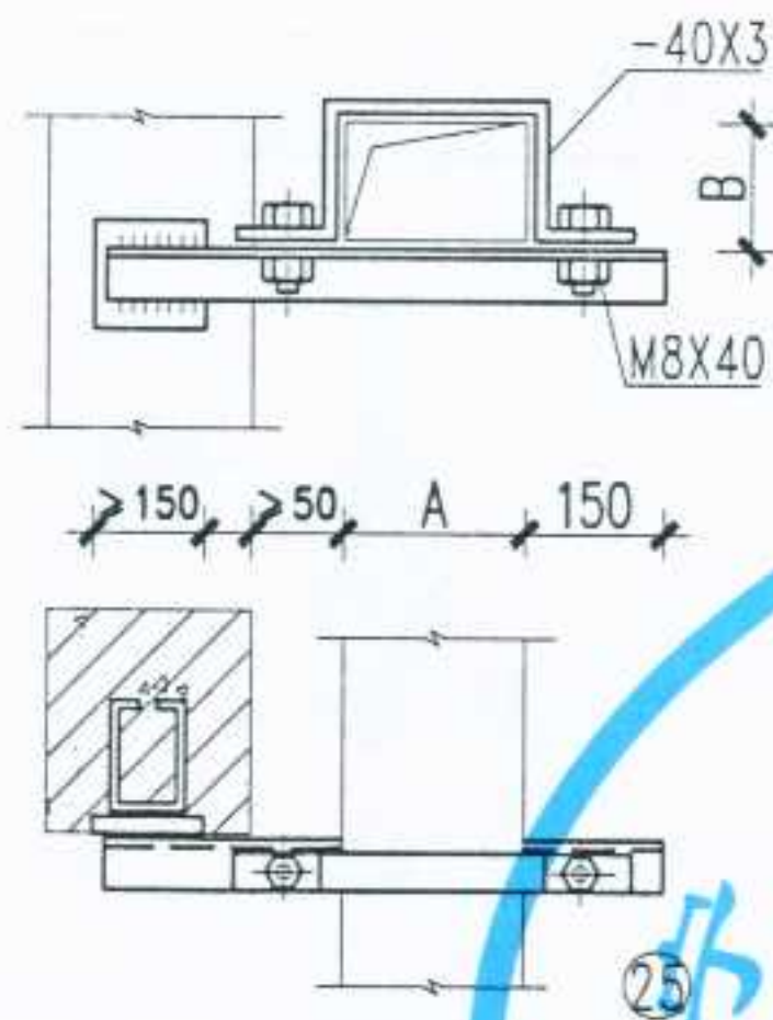
矩形保温风管柱上支架(三)
