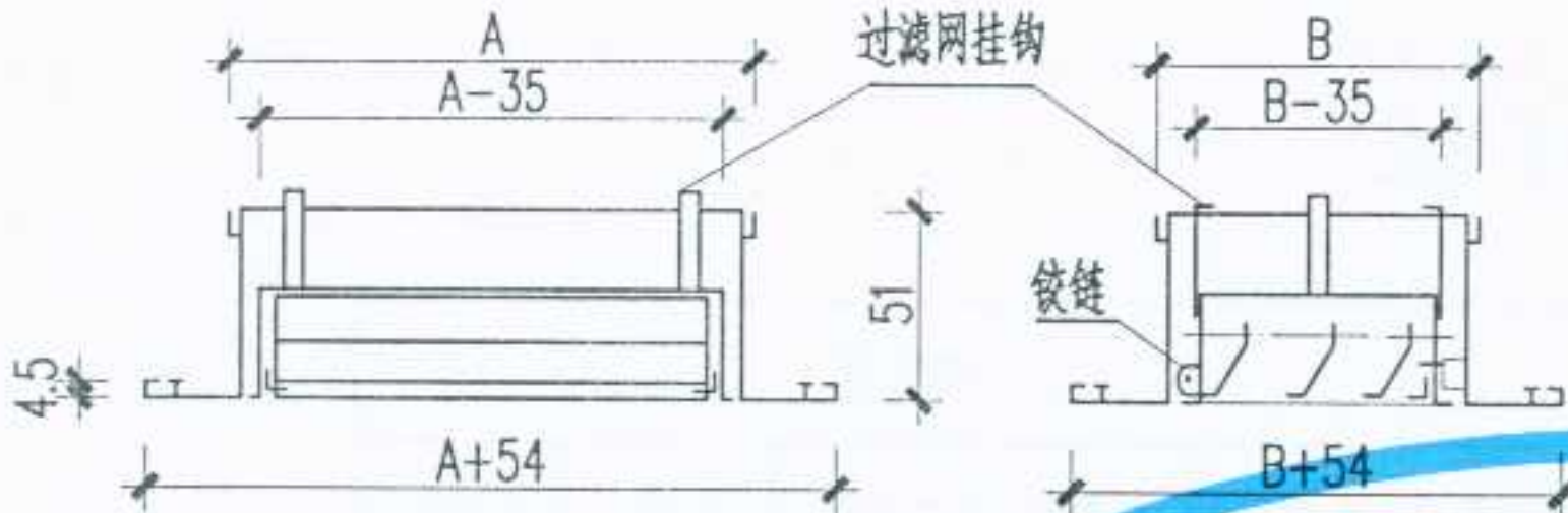
MJ (铝制宽叶片)
