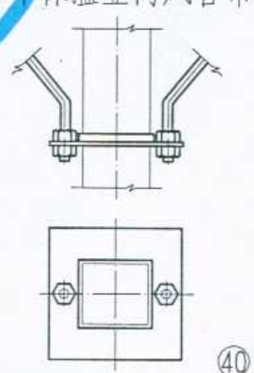
矩形不保温竖向风管吊架
