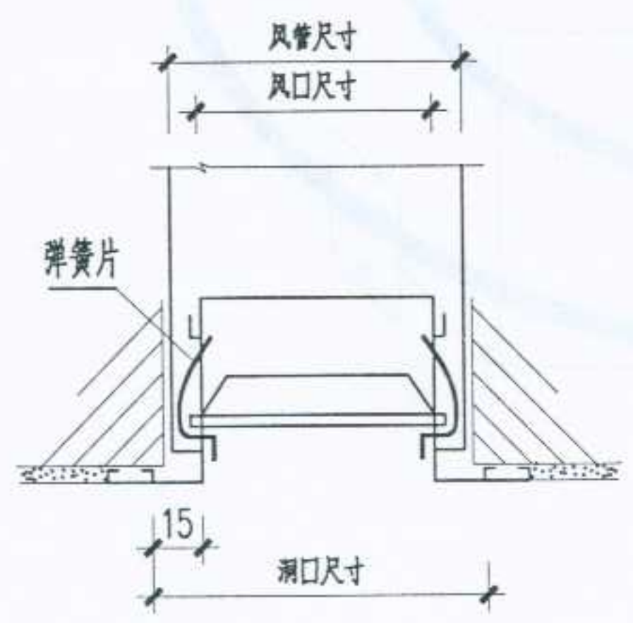
弹簧片安装法
