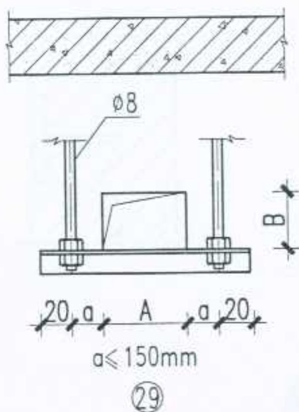
矩形不保温风管双杆吊架
