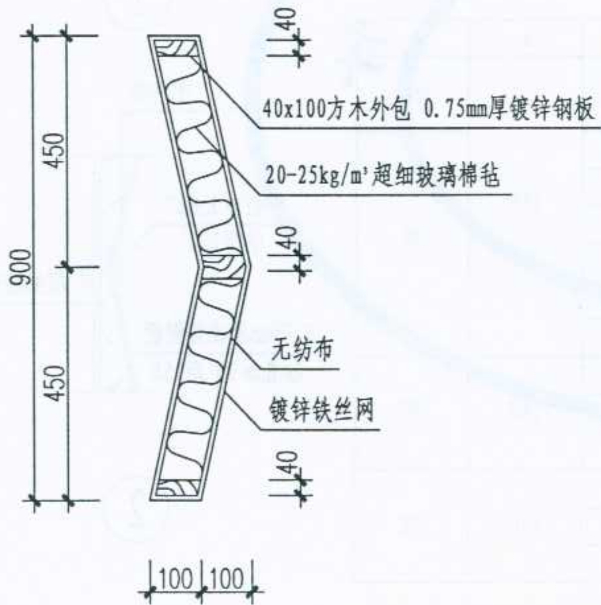
消声片详图
