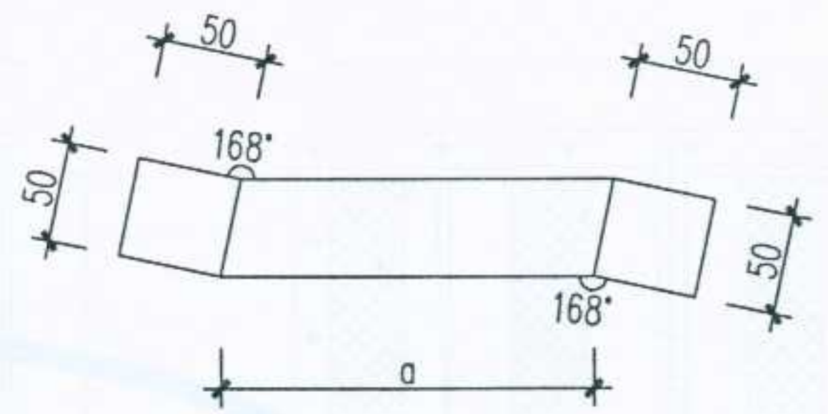
固定卡展开图
