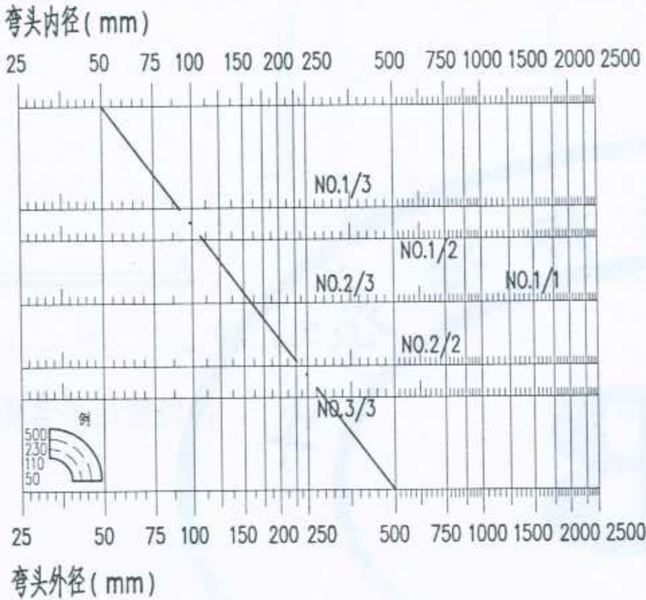
内外弧形矩形弯管内导流叶片设置位置线算图
