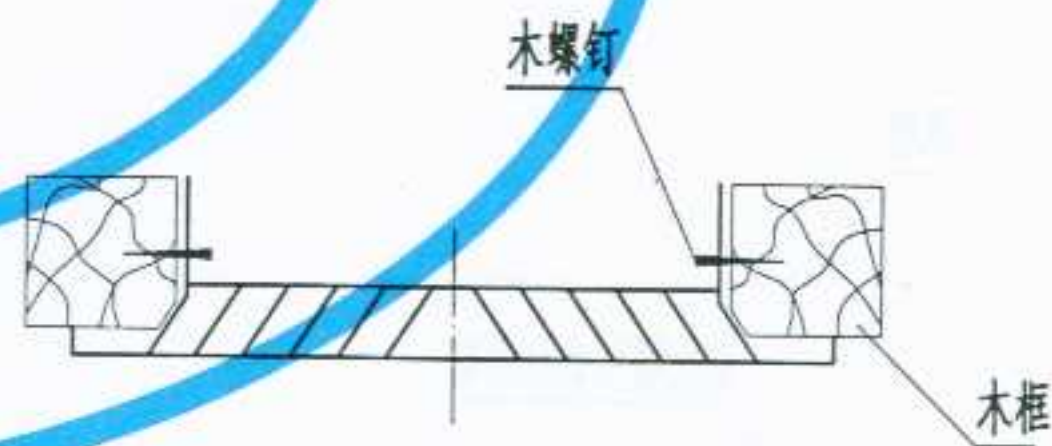
叶片与边框分离式安装法
