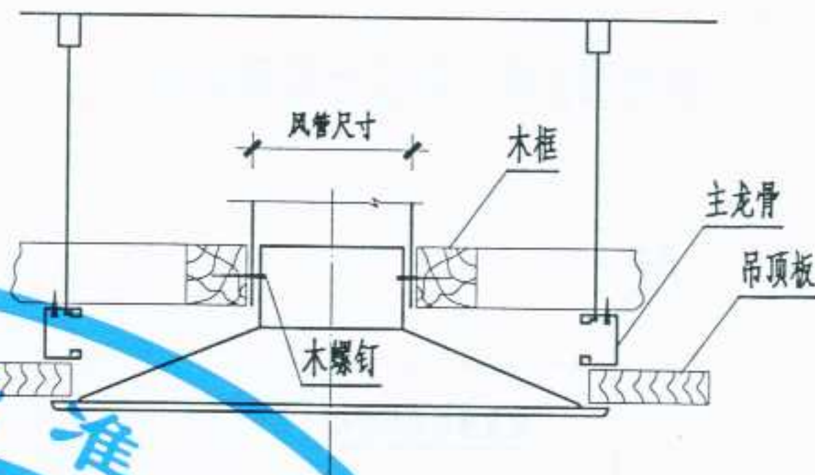
木框设在主龙骨上固定安装法
