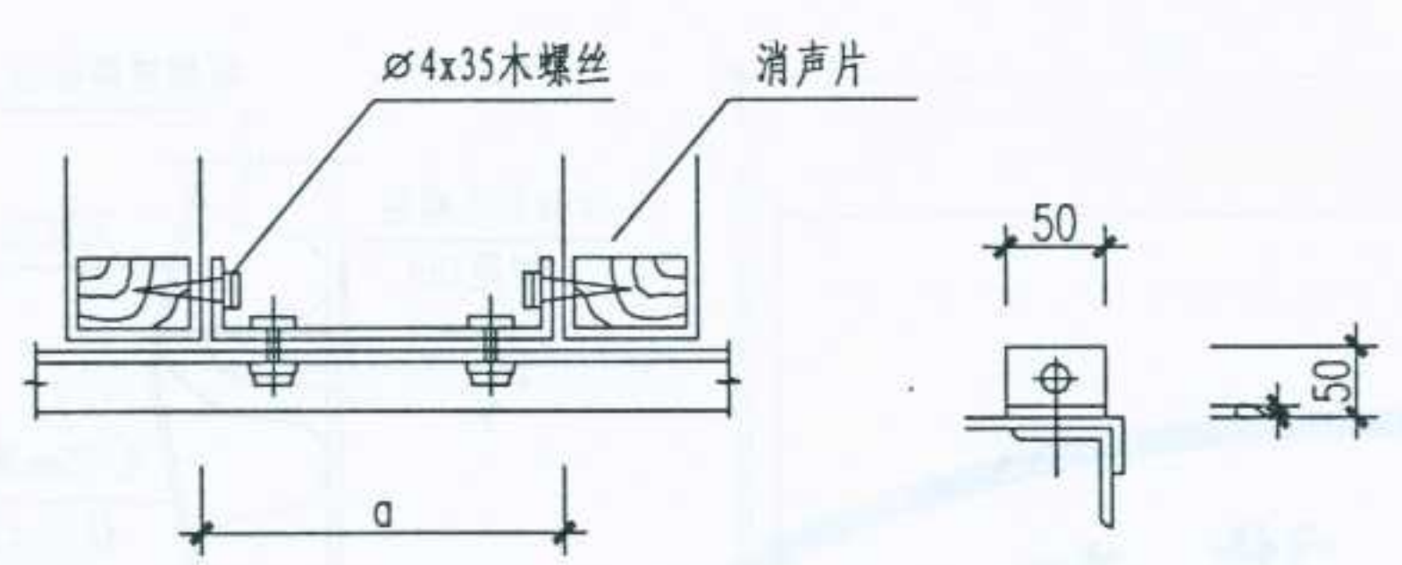
固定卡详图
