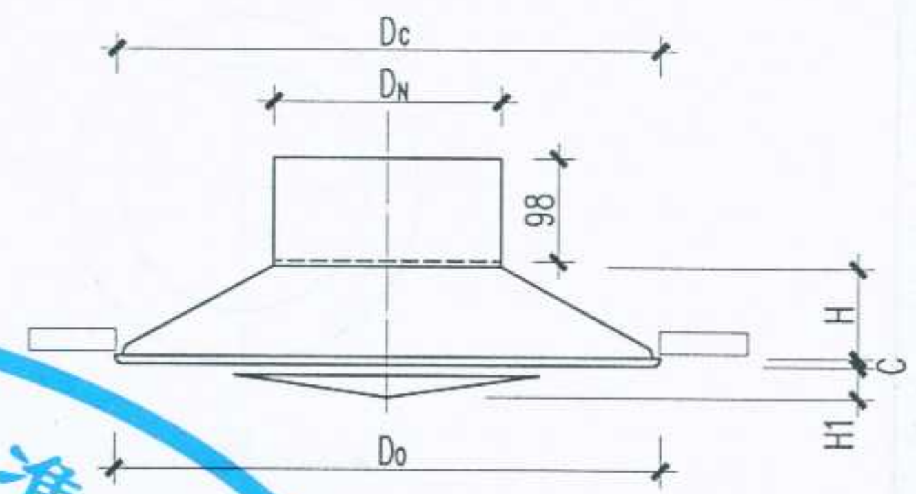
PS (圆盘型)
