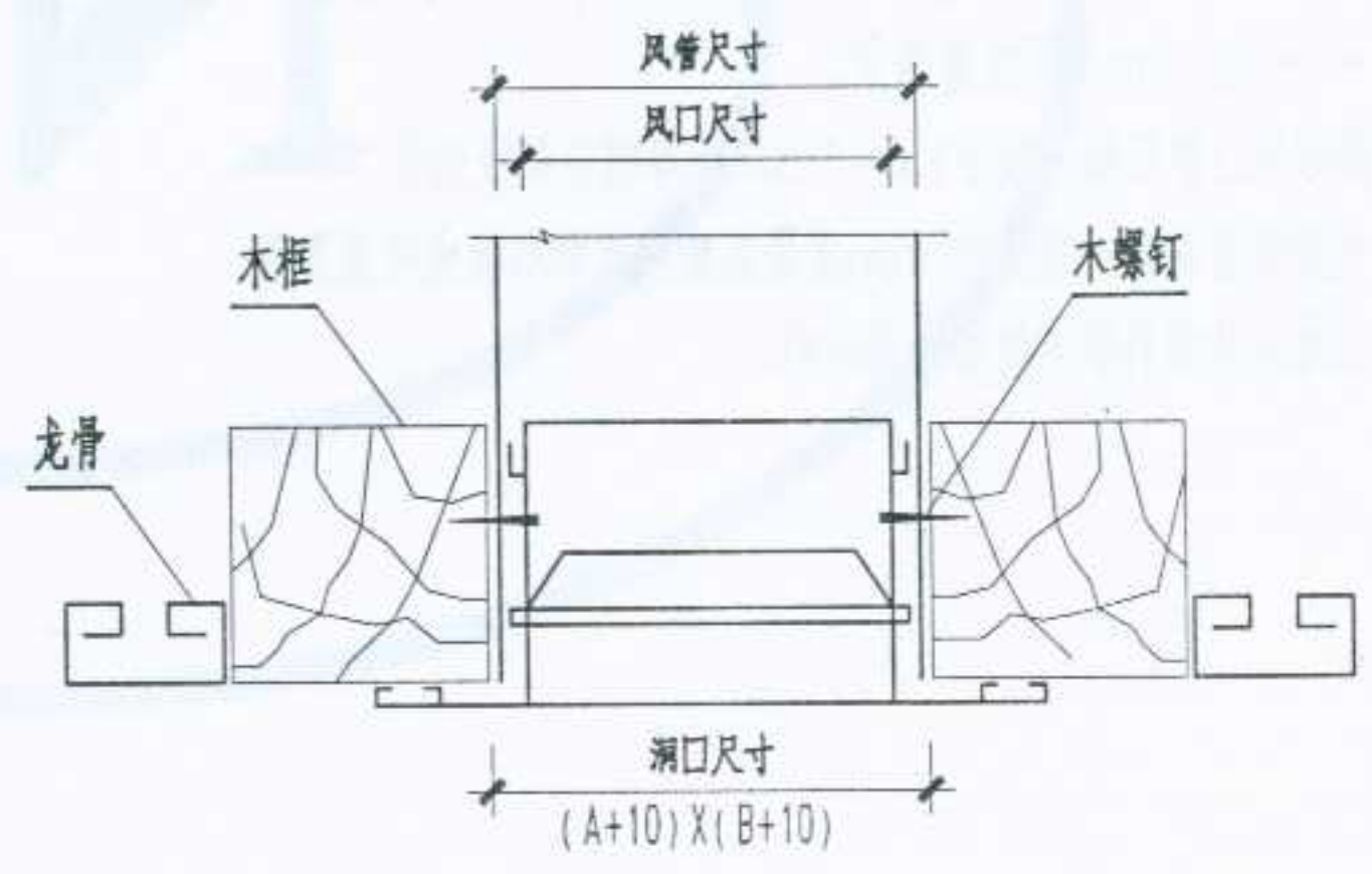
外门框安装法 (二)
