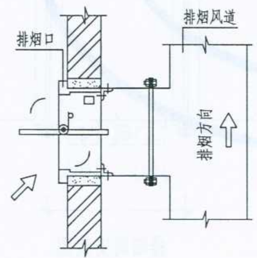
板式排烟口在墙上与铁皮风道安装
