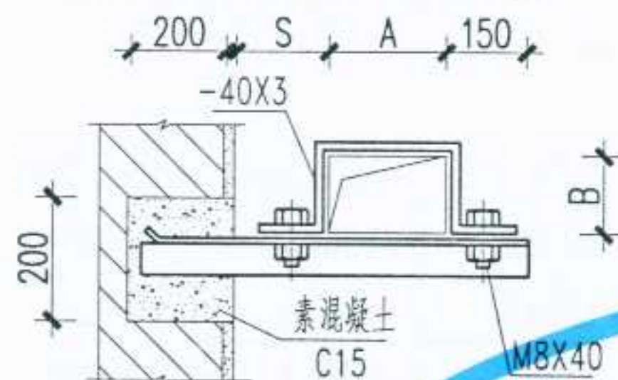
矩形不保温风管墙上支架
