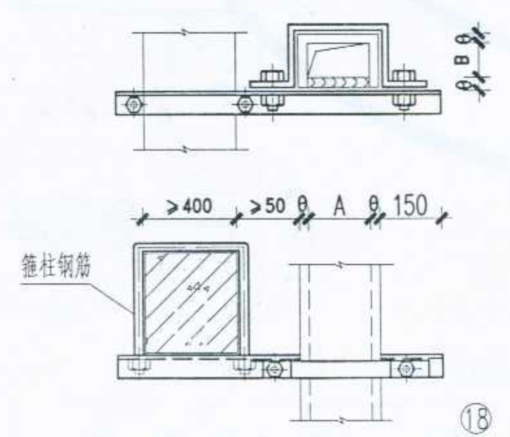
矩形保温风管柱上支架(一)
