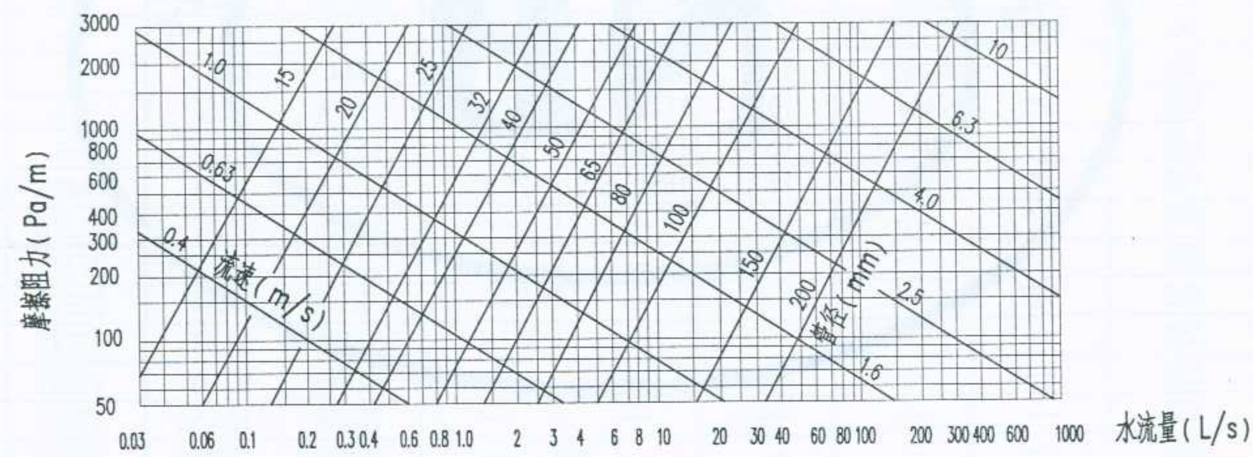
塑料管的水摩擦阻力损失
