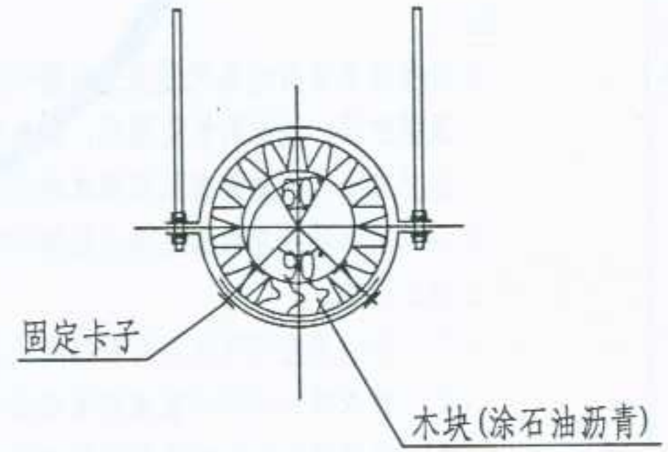
支吊架部位做法
