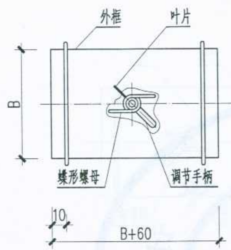
扁形风管小风门
