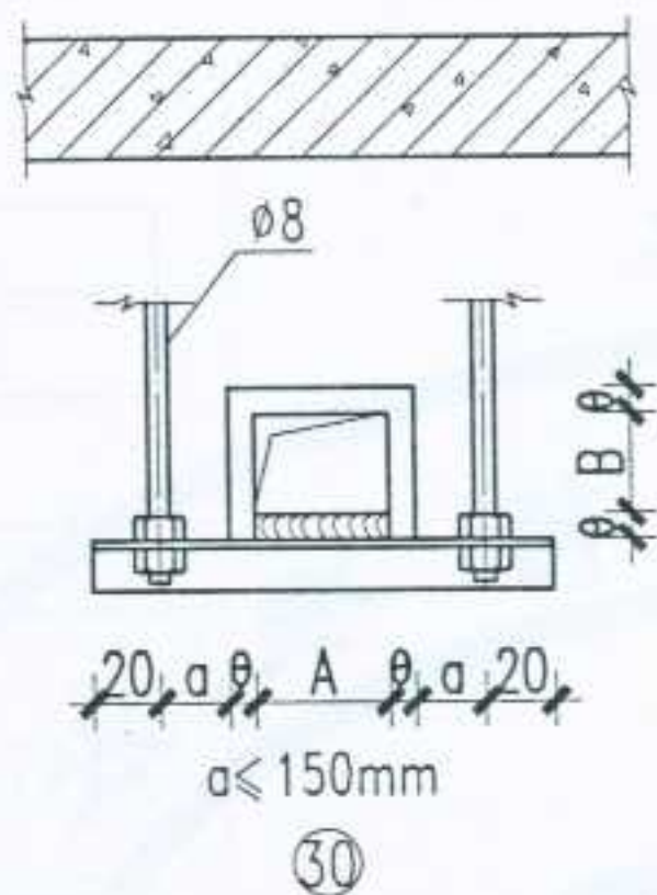
矩形保温风管双杆吊架
