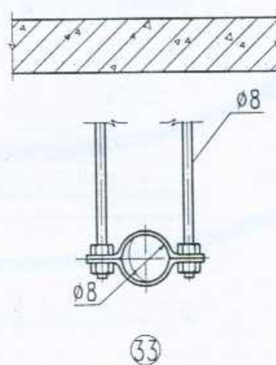
圆形不保温风管双杆吊架
