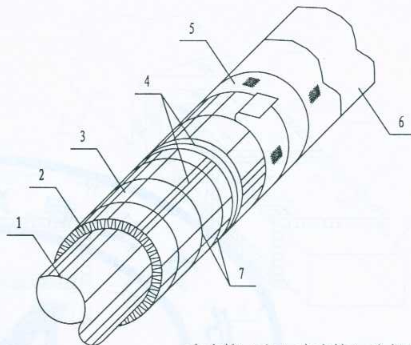
玻璃棉（离心玻璃棉）毡保温
