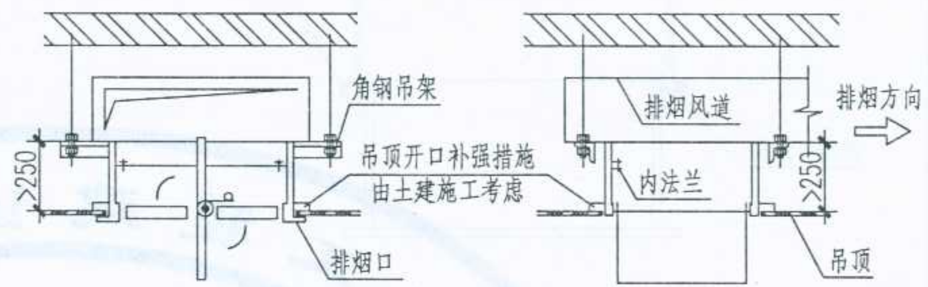
板式排烟口在吊顶上安装
