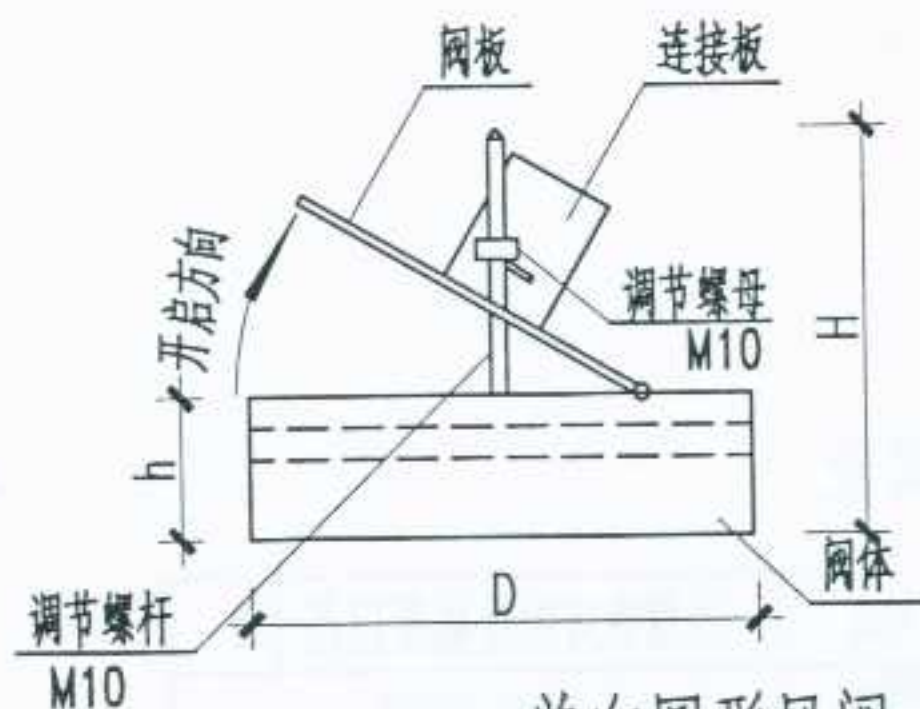
单向圆形风阀
