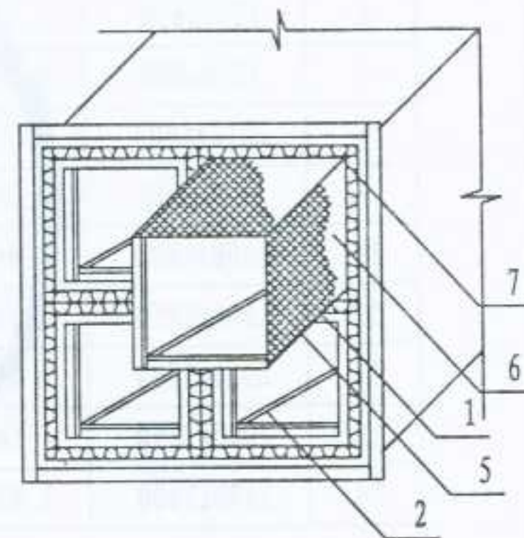
节点构造
