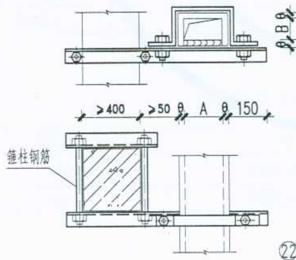
矩形保温风管柱上支架(二)
